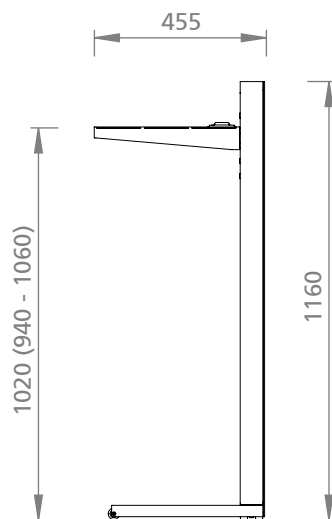
seitenansicht
