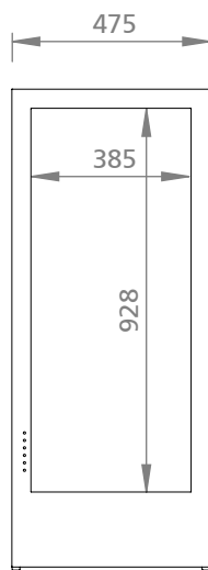
vorderansicht
